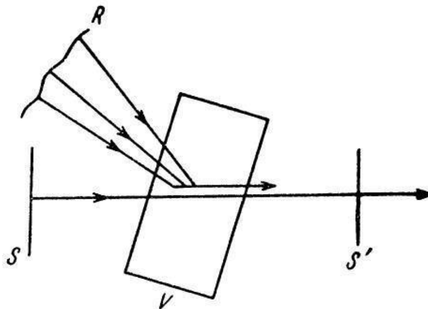
Рис. 2. Коррекция формы волнового фронта излучения лазера с помощью динамической сдвиговой трехмерной голограммы [3].
