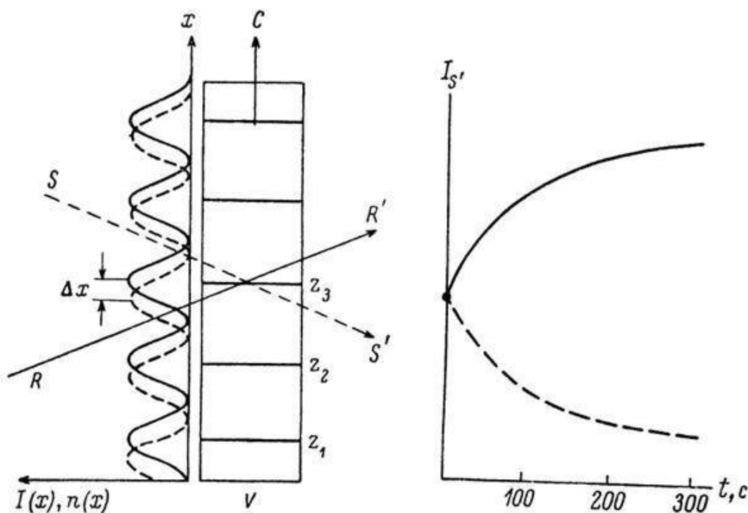
Рис. 1. Схема переноса энергии между объектной и референтной волнами при помощи сдвиговой решетки, возникающей в ниобате лития [3].
